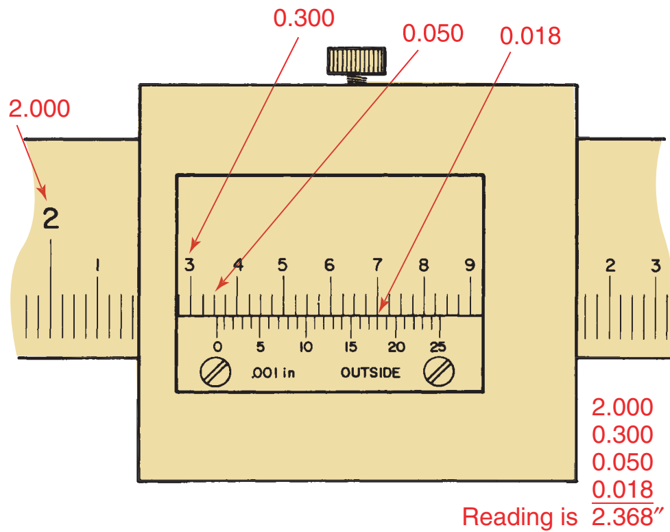
25-Division Vernier
